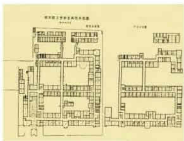
増改築された宇都宮病院平面図
